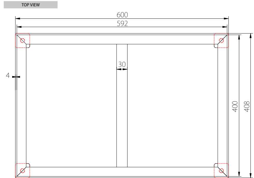
MODEL:SB-D3060/SB-D3973
