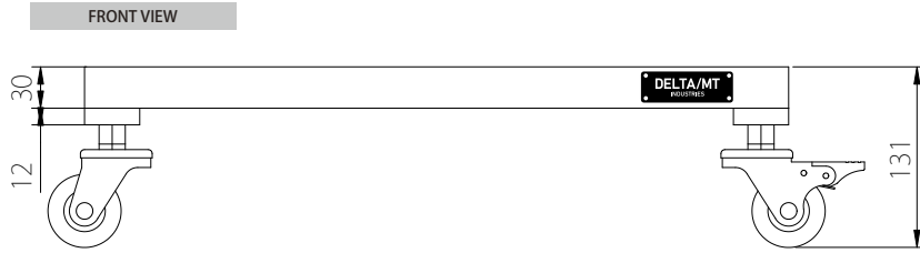
MODEL:SB-D3060
