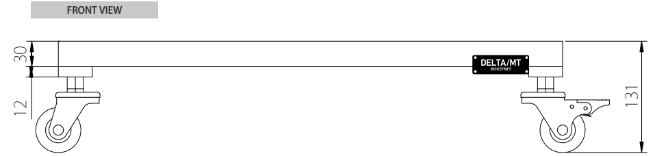
MODEL:SB-D3973
